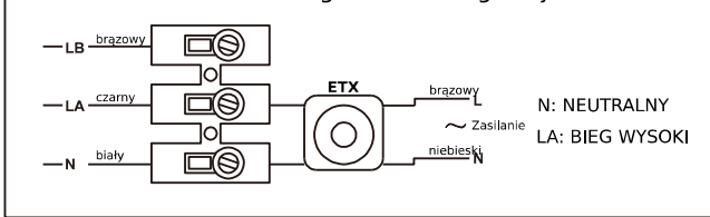
Przełącznik biegów
