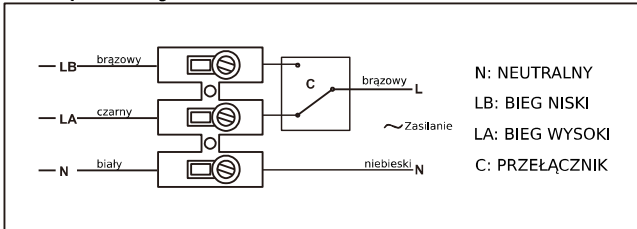
Przełącznik biegów
